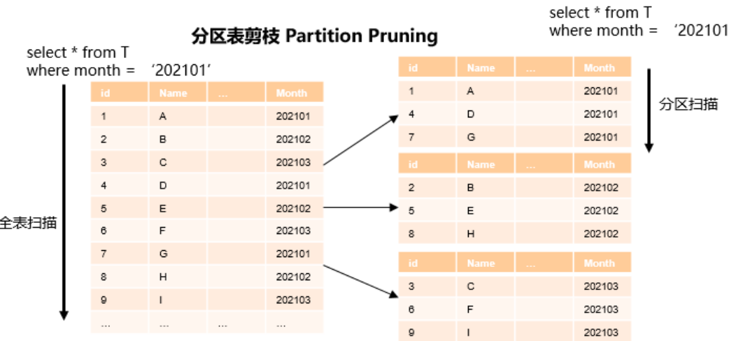
图 8-2 分区表剪枝示例图
