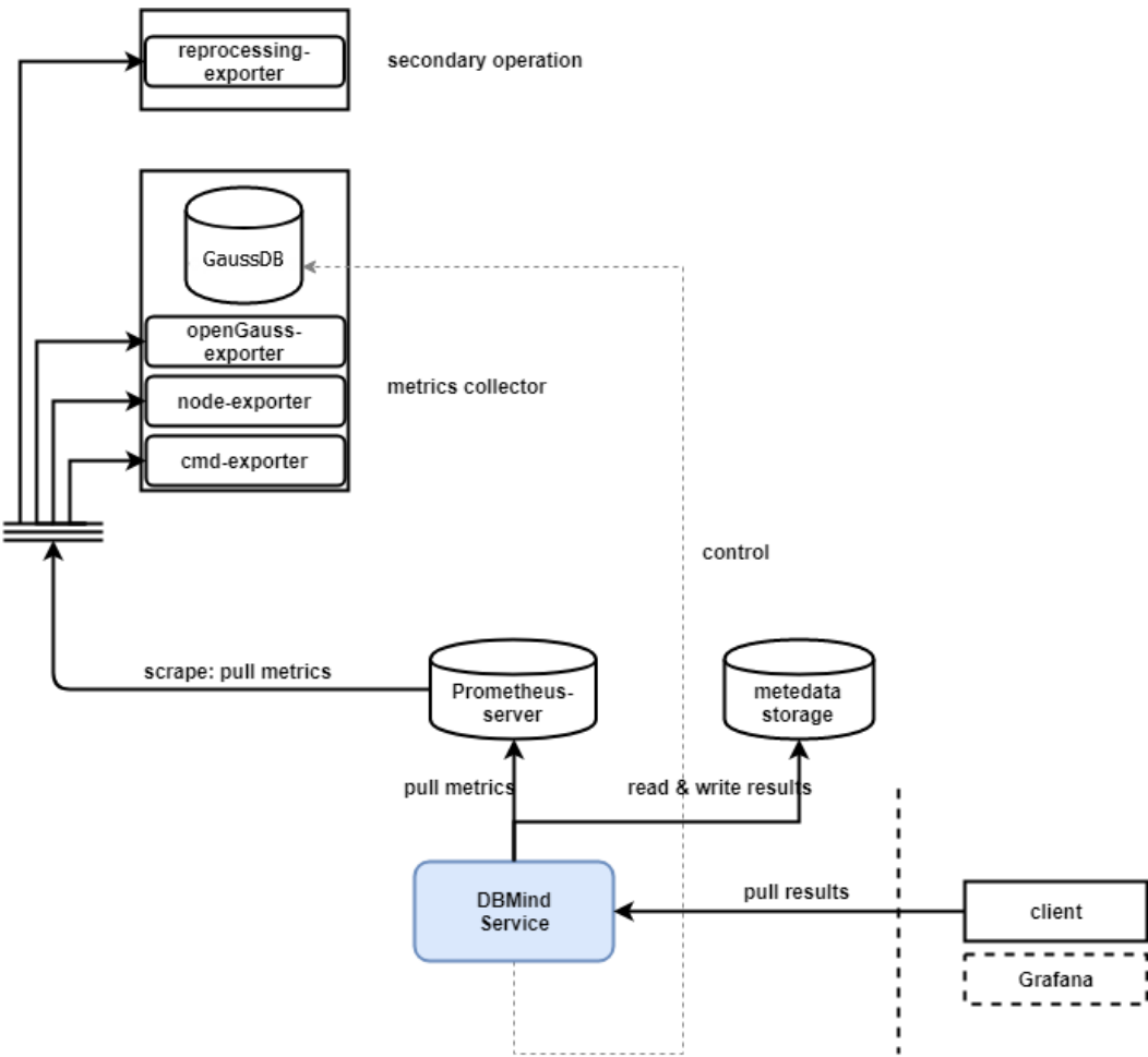
图 11-1 DBMind 服务架构
