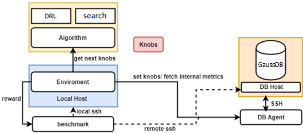
图 11-2 X-Tuner 结构图
