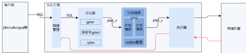
图 15-1 SPM 整体流程
