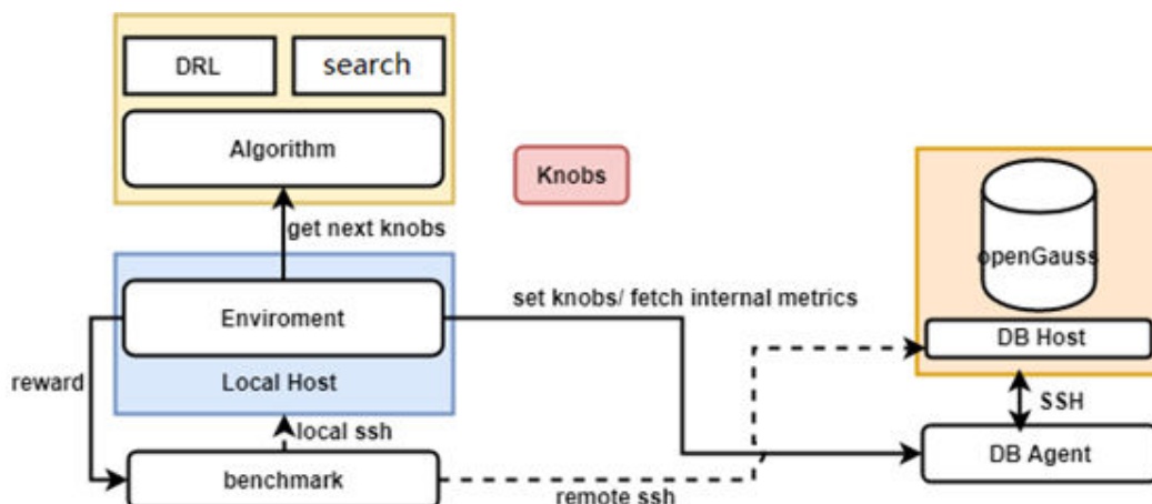
图 10-2 X-Tuner 结构图
